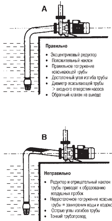
Рис. 1 – Установка насоса
